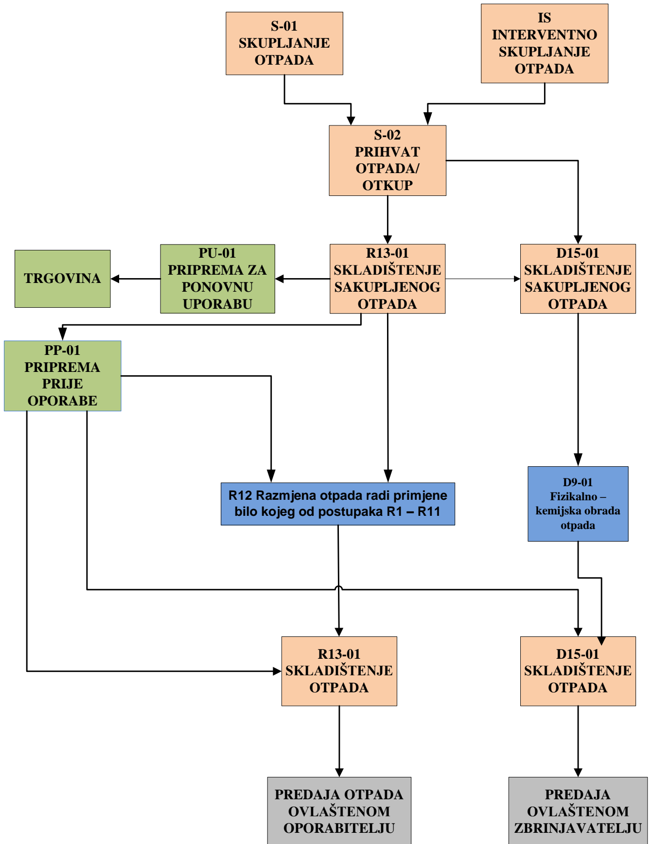
Slika 1. Shematski prikaz tehnoloških procesa
