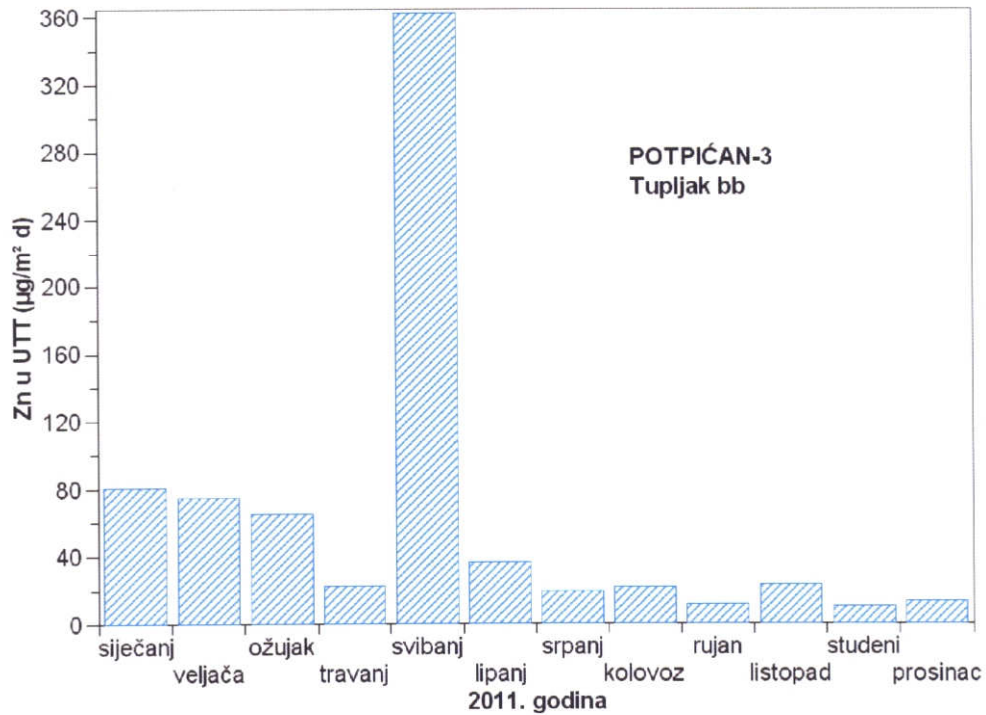
Slika 29 - Srednje mjesečne količine cinka u ukupnoj taložnoj tvari na mjernoj postaji Potpićan-3 tijekom 2011. godine
