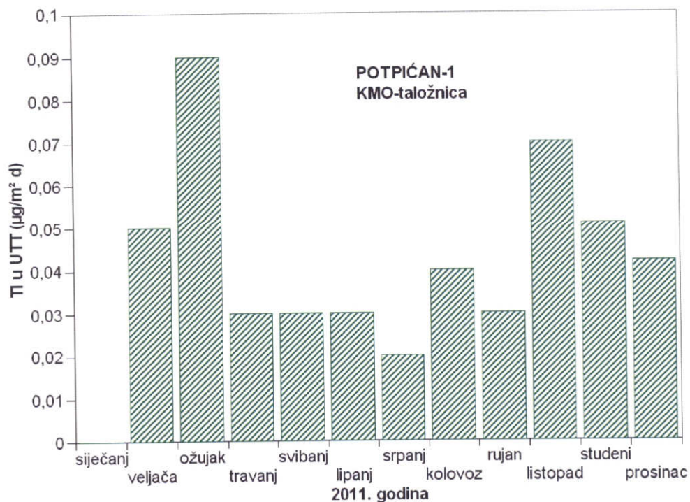
Slika 4 - Srednje mjesečne količine talija u ukupnoj taložnoj tvari na mjernoj postaji Potpićan-1 tijekom 2011. godine
