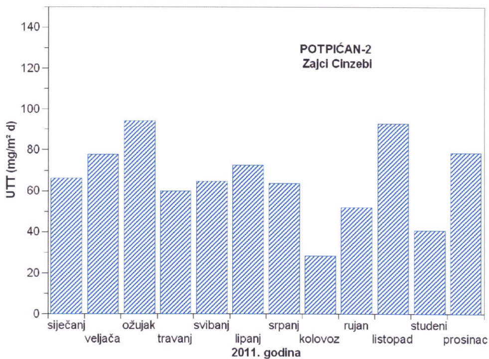
Slika 11 - Srednje mjesečne količine ukupne taložne tvari na mjernoj postaji Potpićan-2 tijekom 2011. godine
