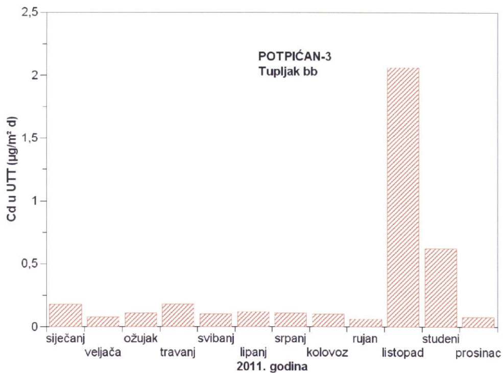
Slika 23 - Srednje mjesečne količine kadmija u ukupnoj taložnoj tvari na mjernoj postaji Potpićan-3 tijekom 2011. godine
