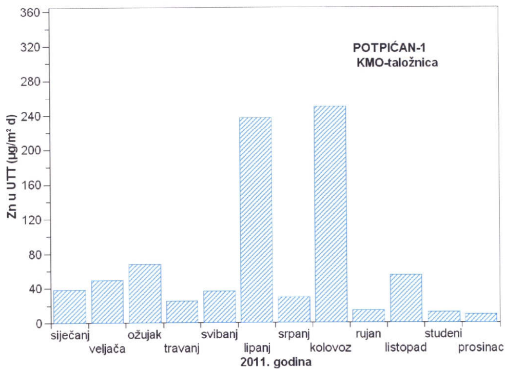
Slika 9 - Srednje mjesečne količine cinka u ukupnoj taložnoj tvari na mjernoj postaji Potpićan-1 tijekom 2011. godine
