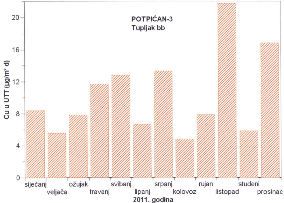
Slika 28 - Srednje mjesečne količine bakra u ukupnoj taložnoj tvari na mjestnoj postaji Potpićan-3 tijekom 2011. godine
