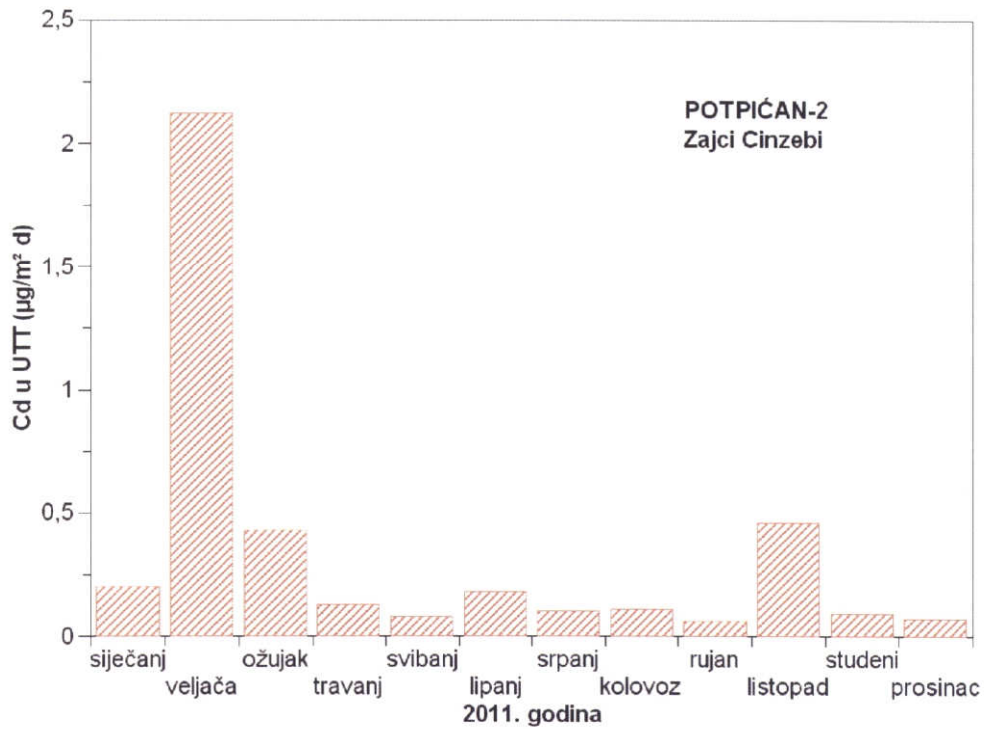
Slika 13 - Srednje mjesečne količine kadmija u ukupnoj taložnoj tvari na mjernoj postaji Potpićan-2 tijekom 2011. godine
