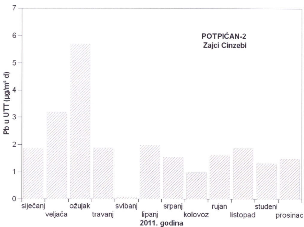
Slika 12 - Srednje mjesečne količine olova u ukupnoj taložnoj tvari na mjernoj postaji Potpićan-2 tijekom 2011. godine
