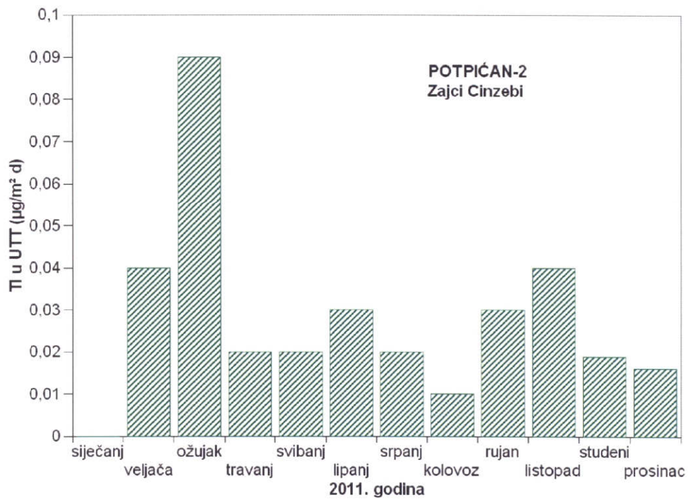
Slika 14 - Srednje mjesečne količine talija u ukupnoj taložnoj tvari na mjernoj postaji Potpićan-2 tijekom 2011. godine
