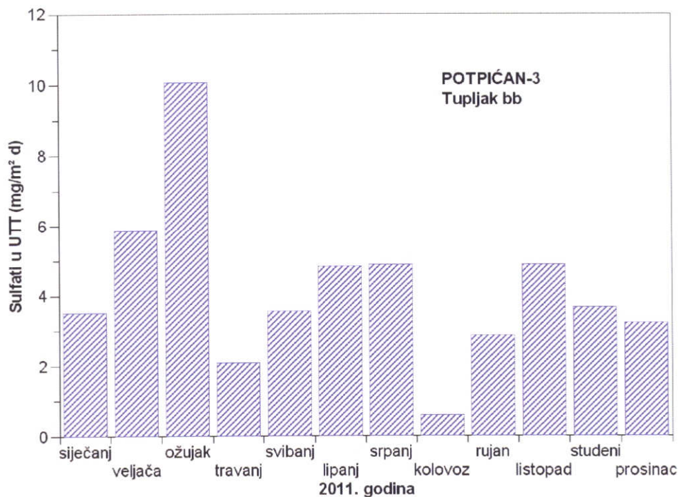
Slika 30 - Srednje mjesečne količine sulfata u ukupnoj taložnoj tvari na mjernoj postaji Potpićan-3 tijekom 2011. godine
