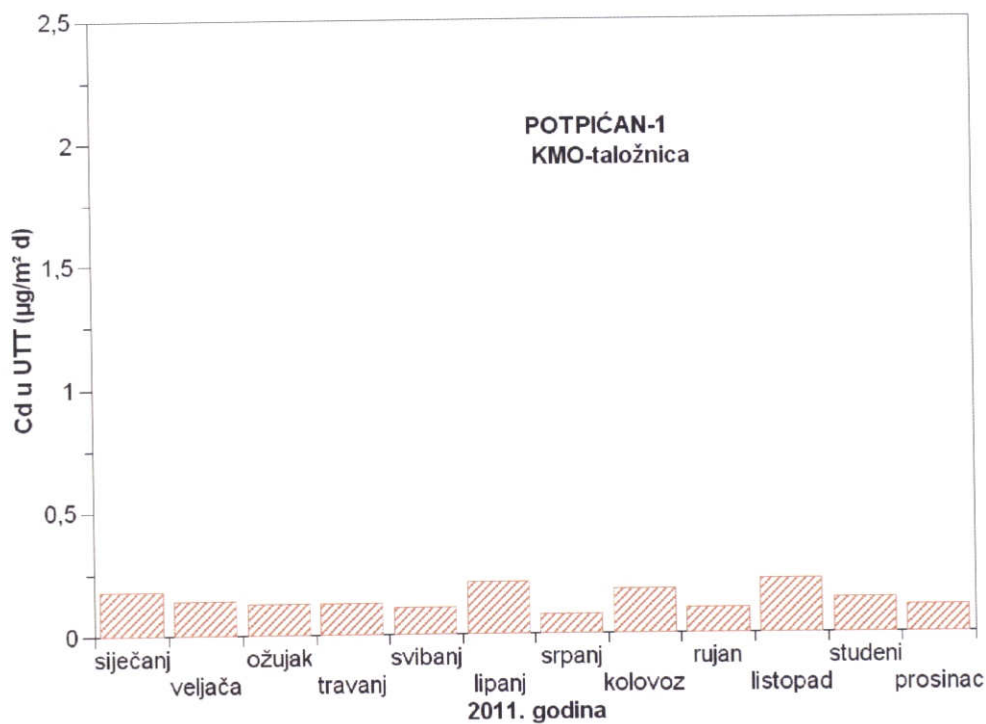
Slika 3 - Srednje mjesečne količine kadmija u ukupnoj taložnoj tvari na mjernoj postaji Potpićan-1 tijekom 2011. godine
