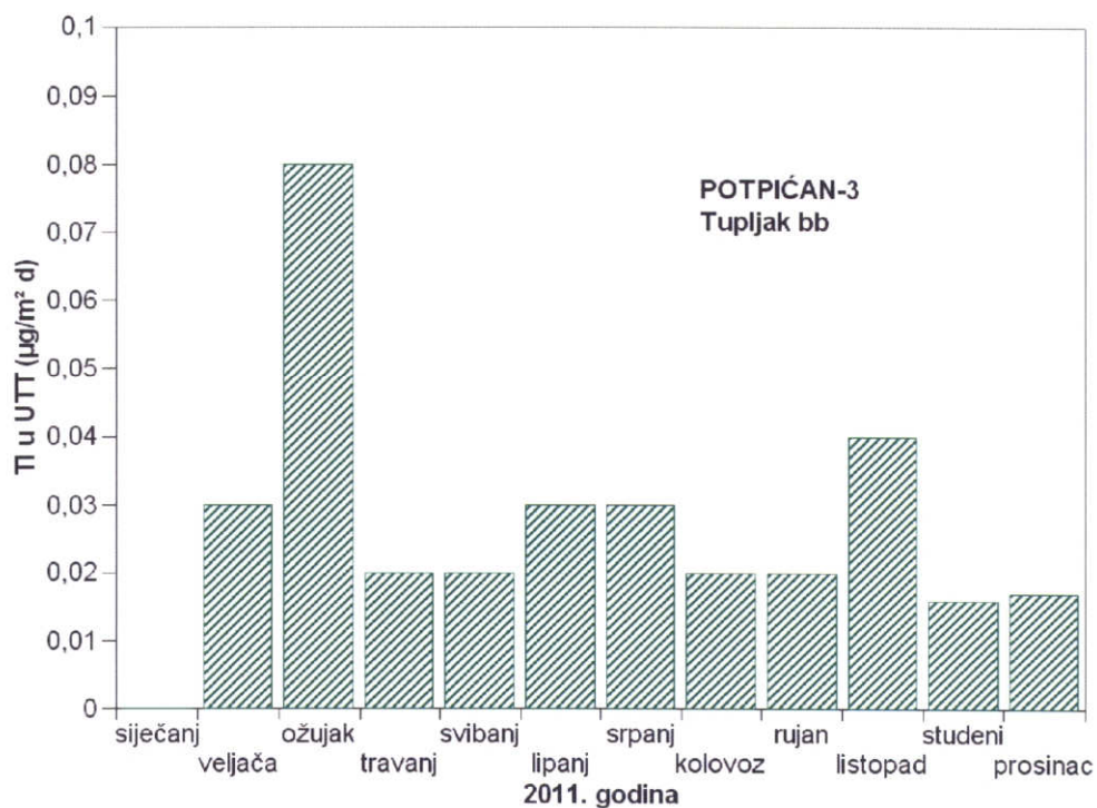
Slika 24 - Srednje mjesečne količine talija u ukupnoj taložnoj tvari na mjernoj postaji Potpićan-3 tijekom 2011. godine
