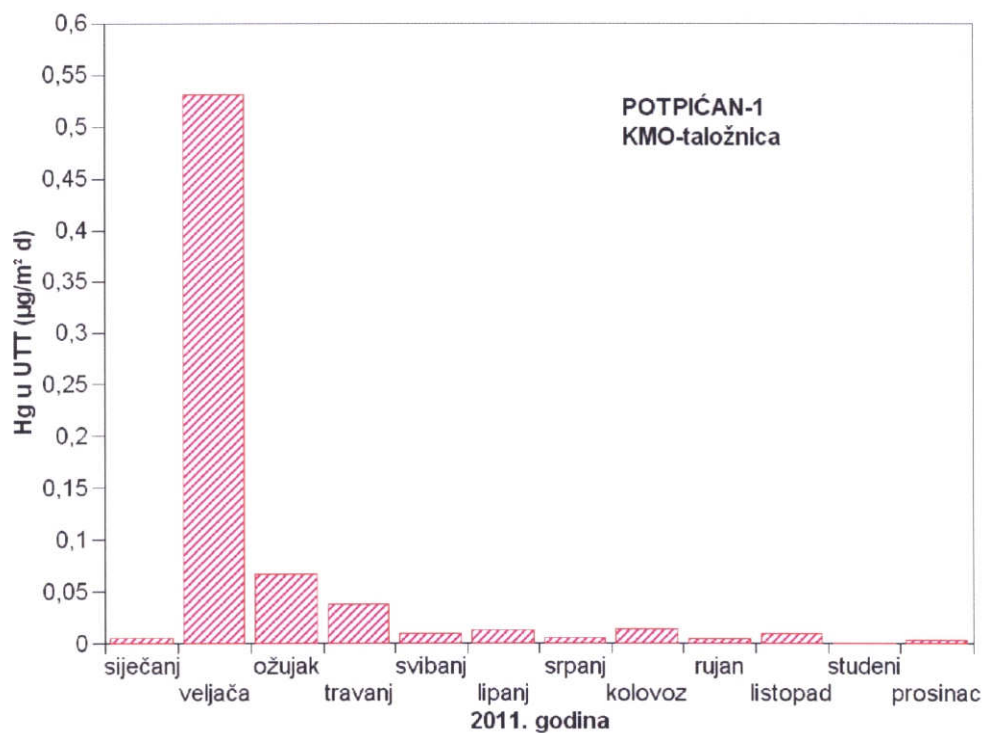
Slika 7 - Srednje mjesečne količine žive u ukupnoj taložnoj tvari na mjernoj postaji Potpićan-1 tijekom 2011. godine
