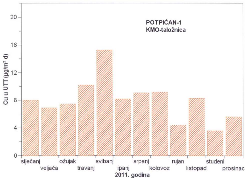
Slika 8 - Srednje mjesečne količine bakra u ukupnoj taložnoj tvari na mjernoj postaji Potpićan-1 tijekom 2011. godine
