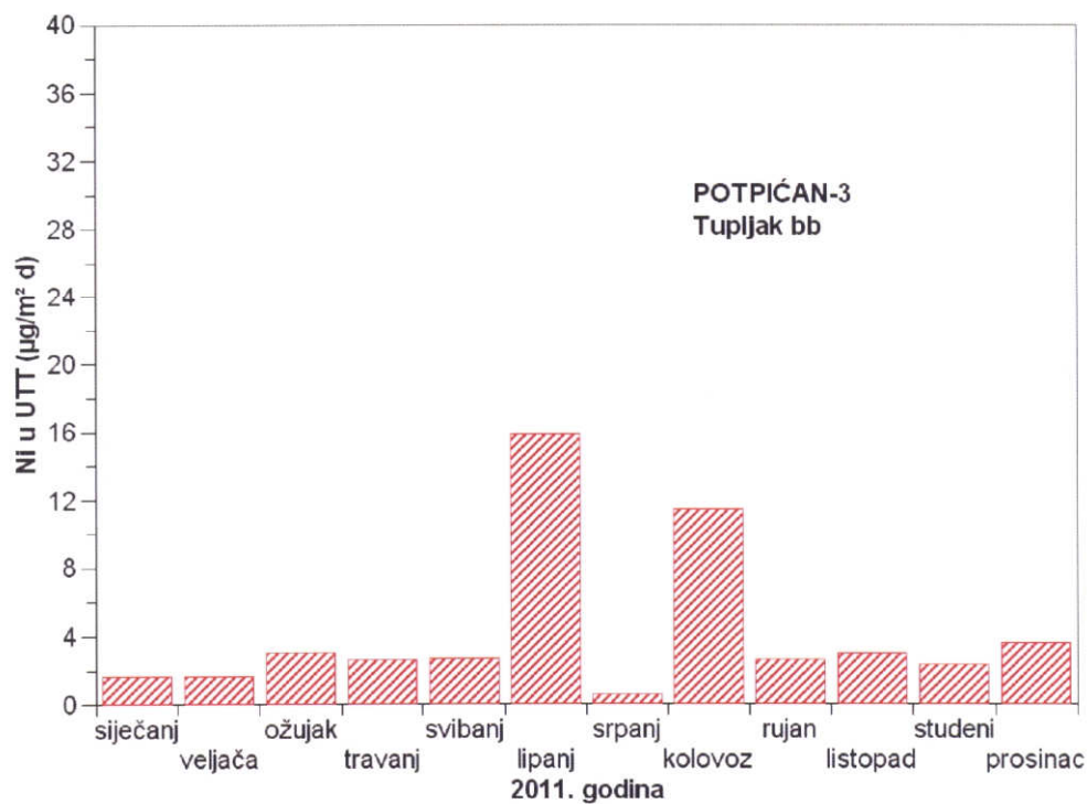
Slika 25 - Srednje mjesečne količine nikla u ukupnoj taložnoj tvari na mjernoj postaji Potpićan-3 tijekom 2011. godine
