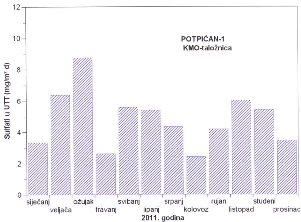
Slika 10 - Srednje mjesečne količine sulfata u ukupnoj taložnoj tvari na mjernoj postaji Potpićan-1 tijekom 2011. godine
