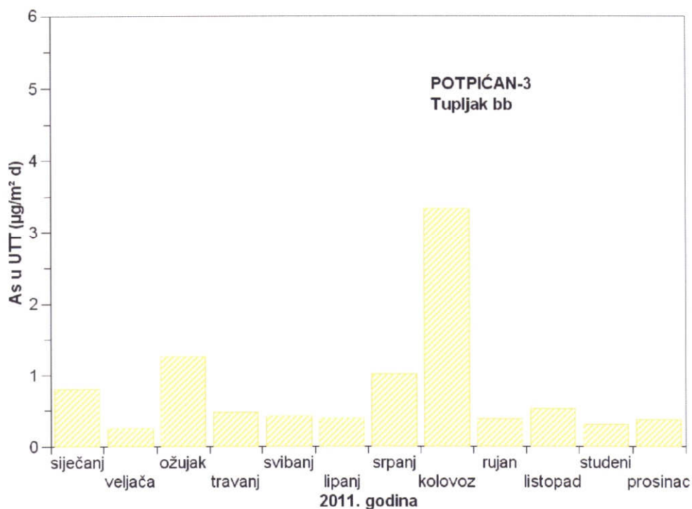
Slika 26 - Srednje mjesečne količine arsena u ukupnoj taložnoj tvari na mjernoj postaji Potpićan-3 tijekom 2011. godine
