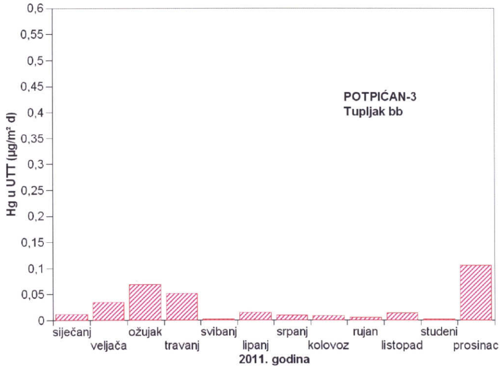
Slika 27 - Srednje mjesečne količine žive u ukupnoj taložnoj tvari na mjestnoj postaji Potpićan-3 tijekom 2011. godine
