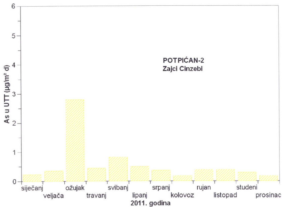
Slika 16 - Srednje mjesečne količine arsena u ukupnoj taložnoj tvari na mjernoj postaji Potpićan-2 tijekom 2011. godine
