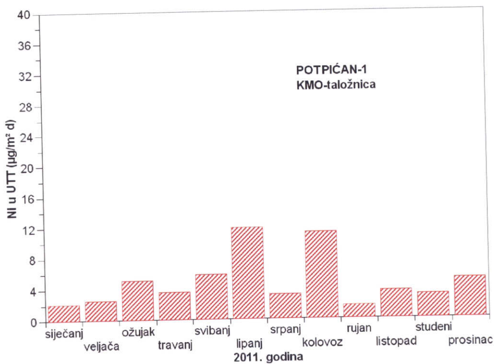
Slika 5 - Srednje mjesečne količine nikla u ukupnoj taložnoj tvari na mjernoj postaji Potpićan-1 tijekom 2011. godine
